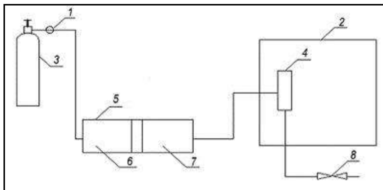
Рис. 2 Схема ввода пробы СУГ в хроматограф 1 - Редуктор; 2 - Хроматограф; 3 - Баллон с рабочим газом; 4 - Система дозирования хроматографа; 5 - Пробоотборник типа ППД; 6 - Камера рабочего газа; 7 - Камера с образцом СУГ; 8 - Запорный вентиль
